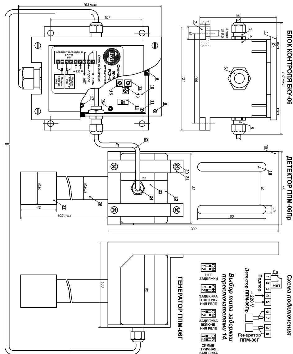
Рис. 1. Сигнализатор уровня РСУ-6.
