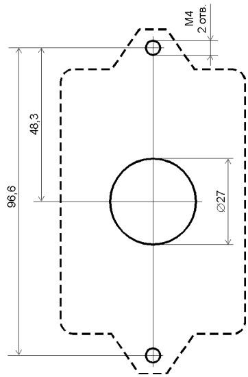
Рис. 3. Отверстия для монтажа модулей МДС-4 и МГ-4.
