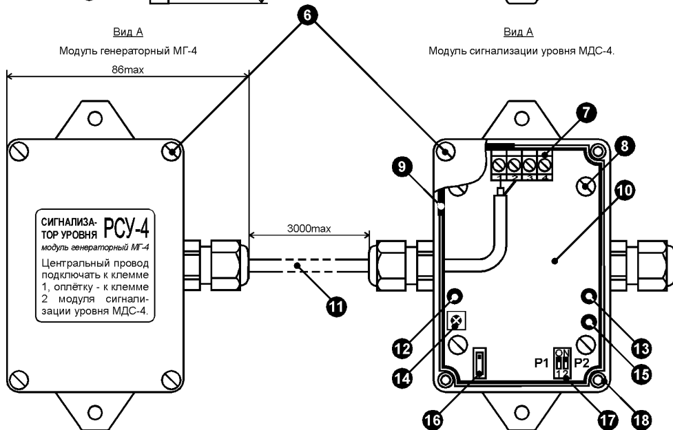
Рис. 2. Конструкция сигнализатора уровня PCSU-4.
