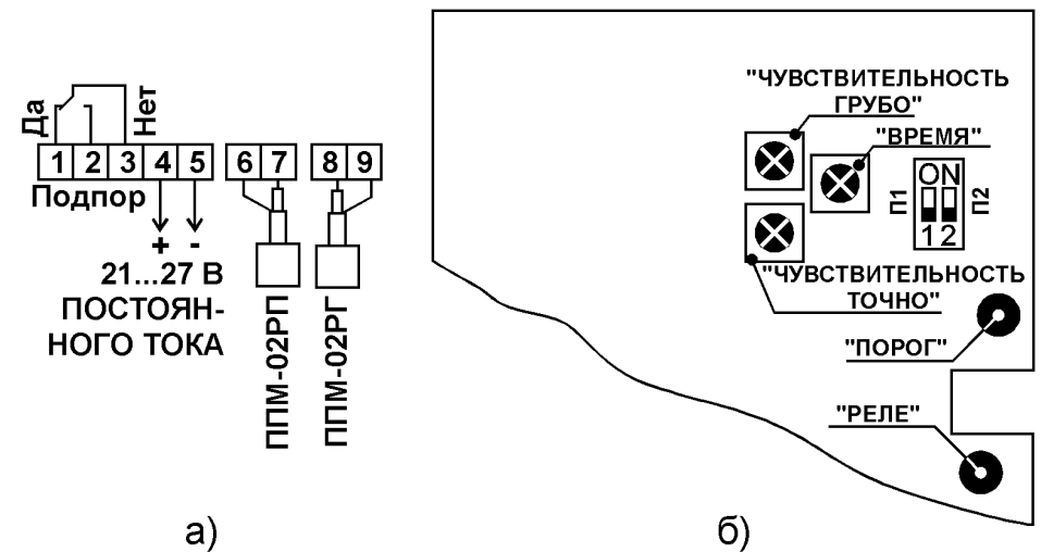
Рис. 8. Схема подключения и органы регулировки датчика РСУ-1РА.
