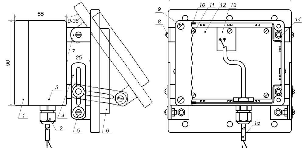
Рис. 5. Конструкция генератора ППМ-02РГ и детектора ППМ-02РП.
