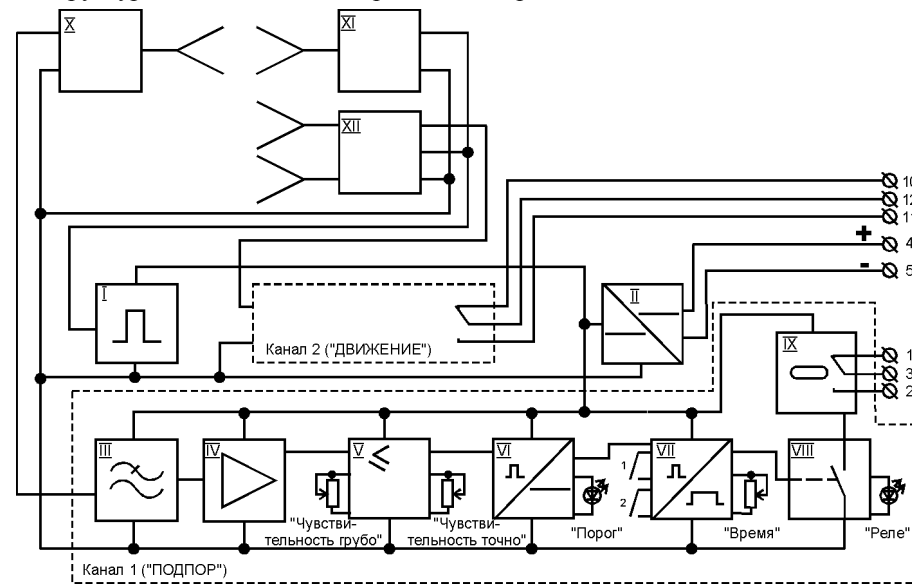
Рис. 5. Структурная схема РДП-02А.
