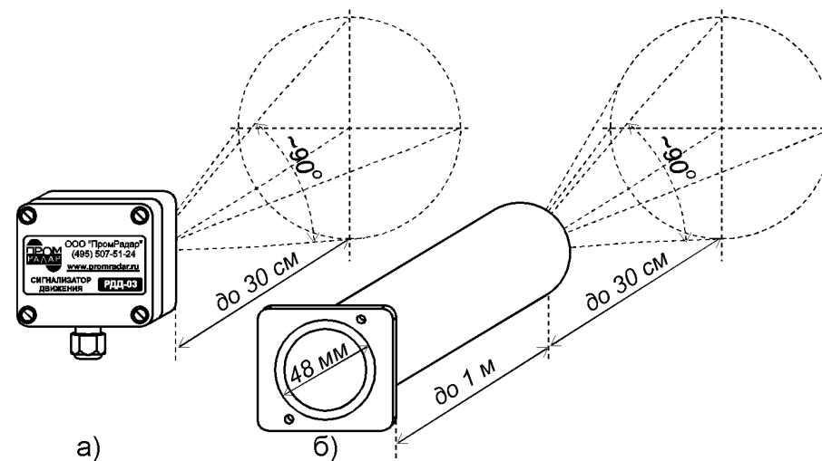
Рис. 3. а) Зона действия датчика. б) Перенос зоны действия с помощью «удлинителя».
