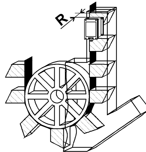
Рис. 3. Контроль сбегания ленты и подпора нории сигнализатором ДС-3А.
