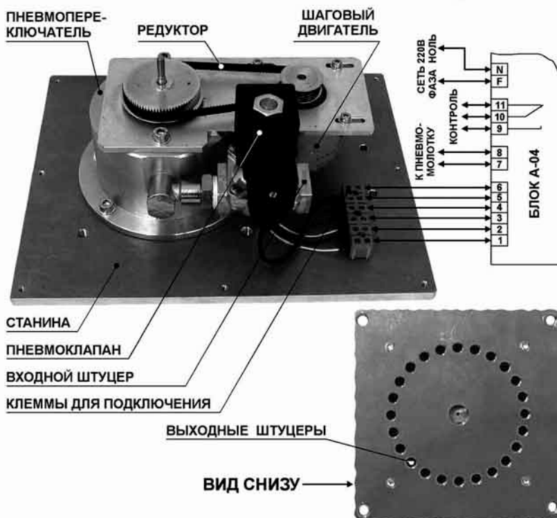
ЭЛЕКТРОМЕХАНИЧЕСКИЙ ПНЕВМОРАСПРЕДЕЛИТЕЛЬ
